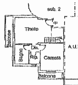
PIANO SECONDO (h. 2,70 m.)
